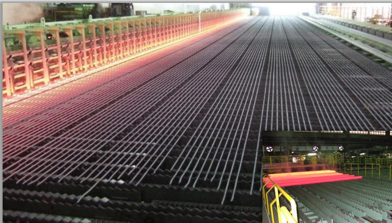
垂直落下式トラフ & 冷却床及び集積コンベア(ランアウトテーブル)
